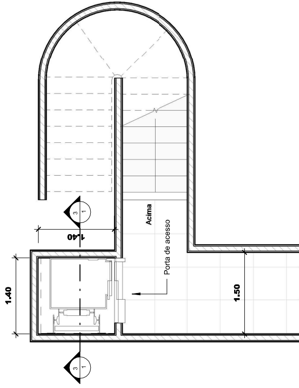
1 Vista Elevador (Térreo)
